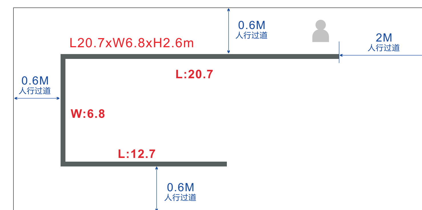
设备占地规划 Machine floor plan:
